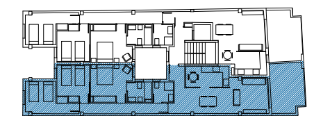
PLANTA ÁTICO
